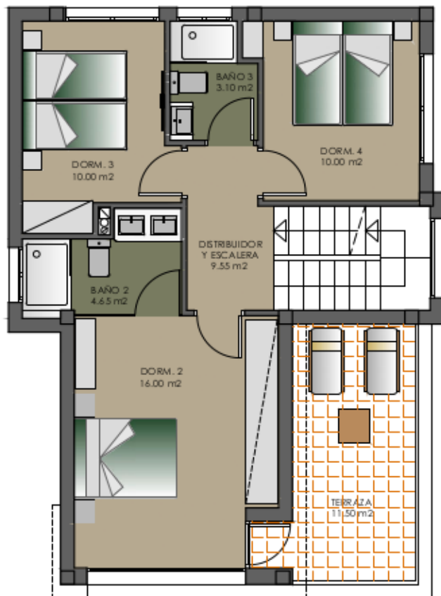
PLANTA PISO
